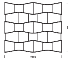
COMPOSIZIONE A / COMPOSITION A L200 P38,5 H173 N. 1_7318 ODX + N. 2_7319 + N.1_7318 OCK + N. 1_7318 OSX
